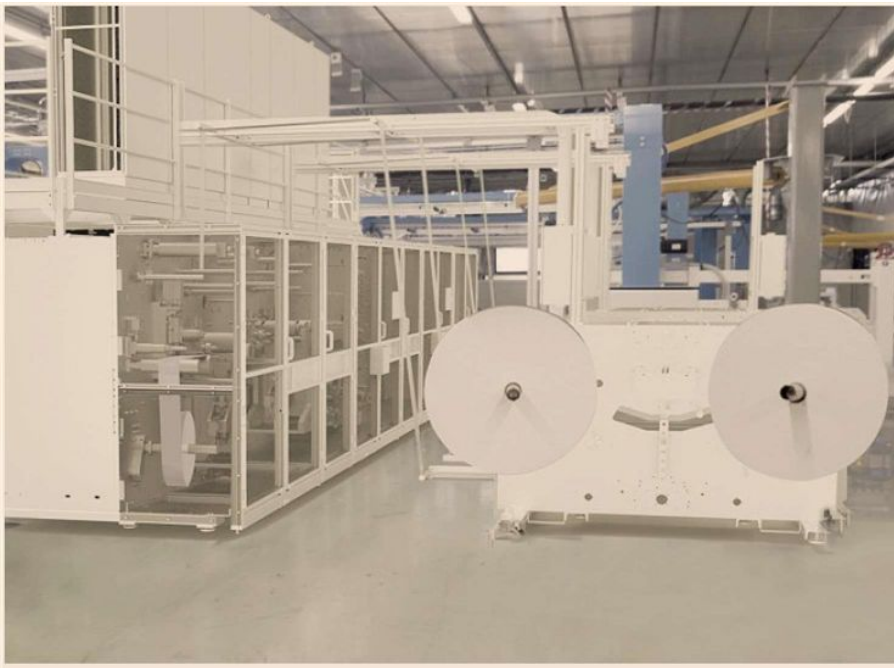
Un milione di pezzi al giorno. La macchina per mascherine più veloce al mondo è stata progettata in Italia dalla Fameccanica e i primi 25 esemplari sono in consegna
