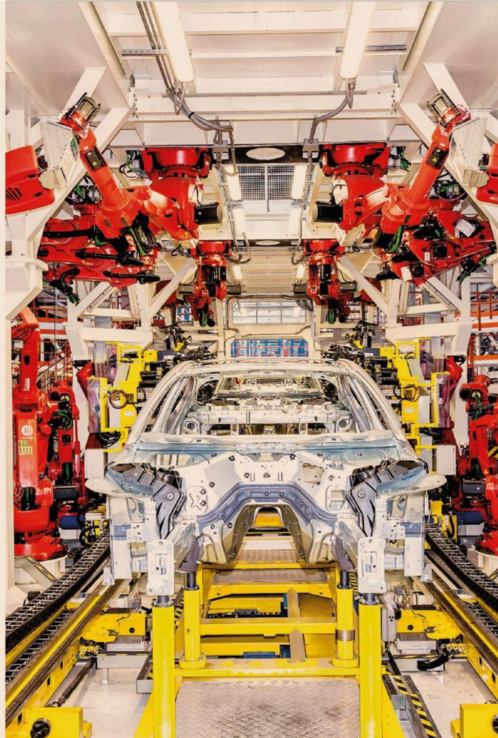
Macchine utensili. Tecnologie e robot Comau installati presso lo stabilimento Fca di Cassino (Frosinone)
