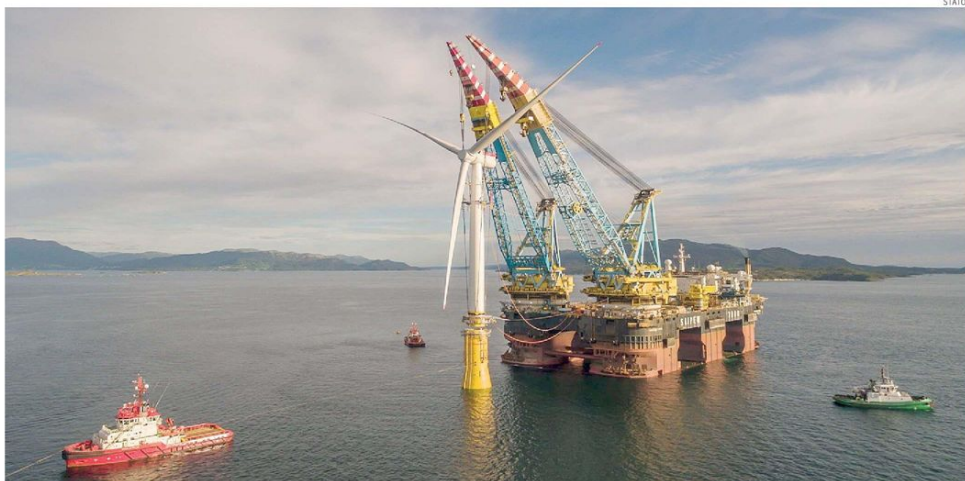
Al largo. La Saipem 7000 durante la posa dei colossali generatori eolici del progetto hywind . Sotto, a sinistra, fervono i lavori sul ponte di coperta della Saipem 7000: sul lato destro, è posata una piccola pala, lunga una quarantina di metri, da installare su un "ventilatore" eolico. Sotto, a destra, il ponte di comando della nave, con in primo piano i quadri di comando delle zavorre
