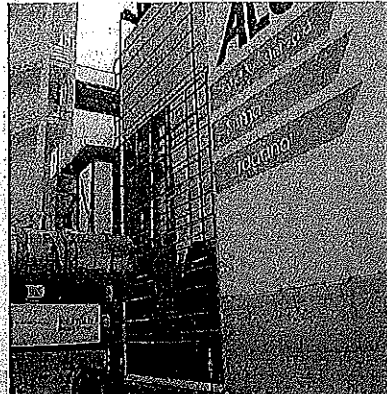
La torre. La struttura alta 16 metri su cui effettuare test sugli elementi costruttivi alle condizioni di rischio ambientale e sismico
