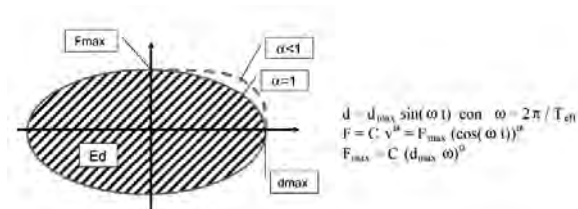
Fig. 11.9.2 – Dispositivi a comportamento viscoso
