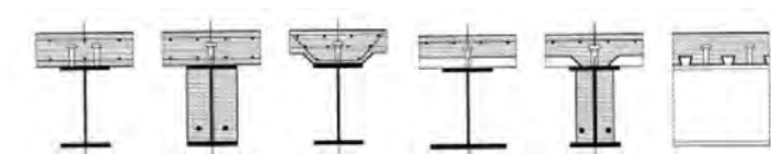
Fig. 4.3.3 - Tipologie di sezione composte per travi
