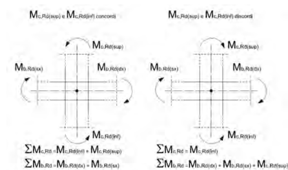
Fig. 7.4.2 – Progettazione in capacità dei pilastri
