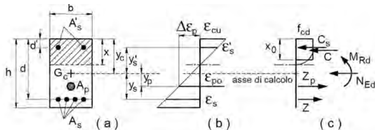
Fig. 4.1.4 - Sezione pressoinflessa
