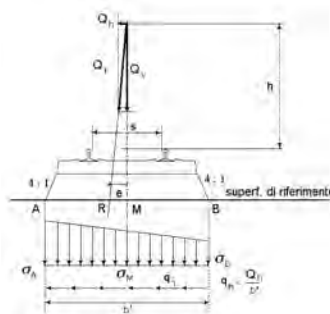
Fig. 5.2.5 - Distribuzione trasversale in rettifilo delle azioni per mezzo delle traverse e del ballast. In figura, Q_n rappresenta la forza centrifuga definita al successivo §5.2.2.3.1
