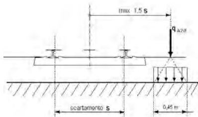
Fig. 5.2.13 - Caso 2
